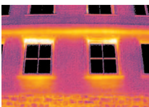
Демонстрация тепловых потерь при неправильной изоляции радиаторных ниш
