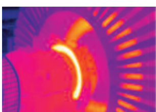
Проверка состояния механических деталей (подшипников и валов) на предмет неполадок
